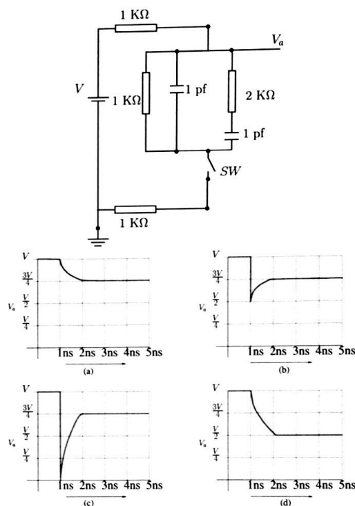
FIGURE 3 – Circuit RC et propositions de courbe pour la tension V(a) .
